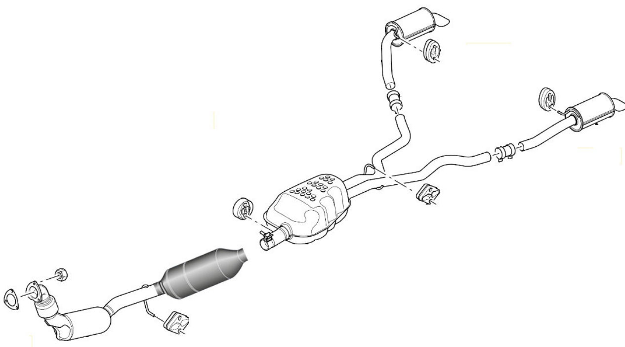
Partikelfilteret monteres imellem ophæng og mellempotte.
