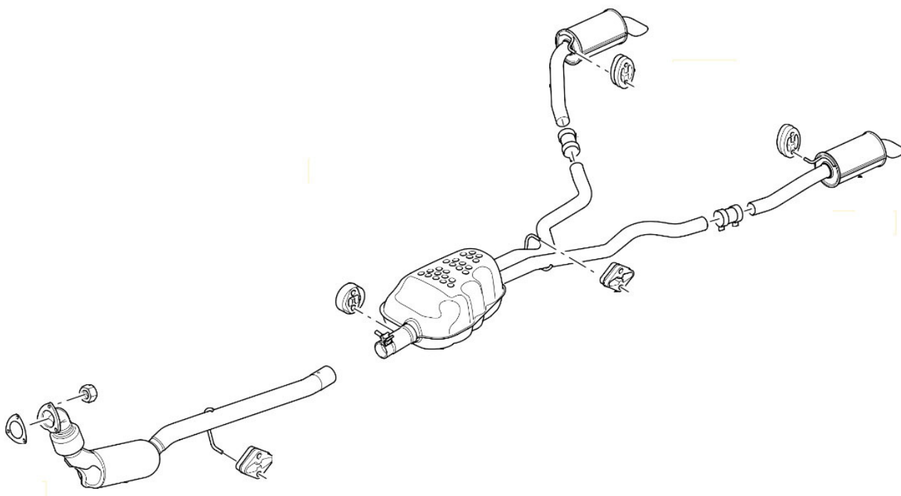
Original udstødning, fra venstre : Forrør katalysator, mellempotte og 2 bagpotter.
